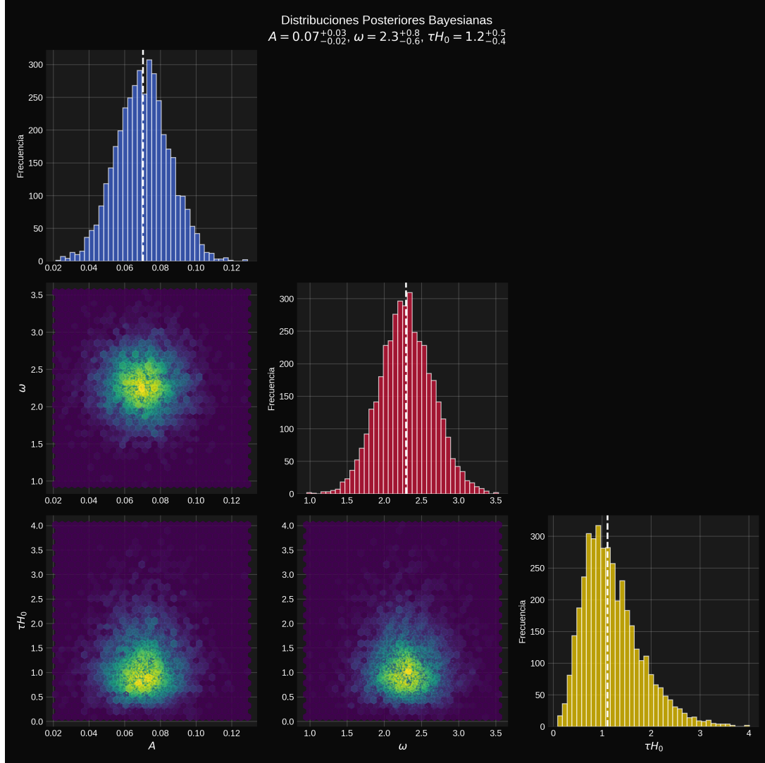
Figura 4: Distribuciones posteriores bayesianas para los parámetros (A, \omega, \tau) . Los contornos de densidad y las distribuciones marginales confirman: A = 0,07^{+0,03}_{-0,02} , \omega = 2,3^{+0,8}_{-0,6} , \tau H_0 = 1,2^{+0,5}_{-0,4} .
