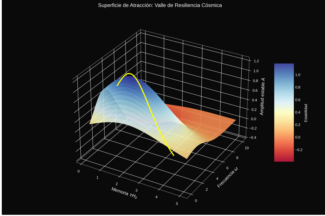
Figura 3: Superficie de atracción mostrando regiones estables (azul) e inestables (rojo). El valle diagonal dorado representa la banda de resiliencia cósmica donde la memoria ( \tau ) y la frecuencia ( \omega ) permiten oscilaciones sostenidas.
