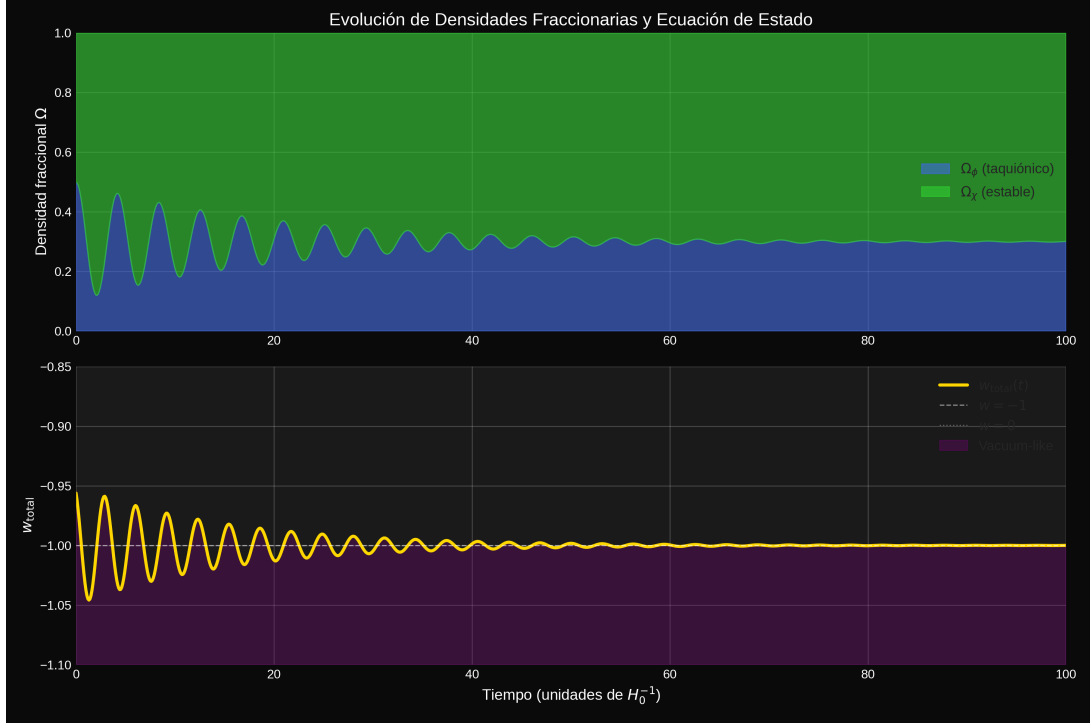
Figura 5: Panel superior: evolución de las densidades fraccionarias mostrando intercambio de energía entre los campos taquiónico y estable. Panel inferior: la ecuación de estado total exhibe oscilaciones alrededor de w = -1 con fases vacuum-like dominantes.
