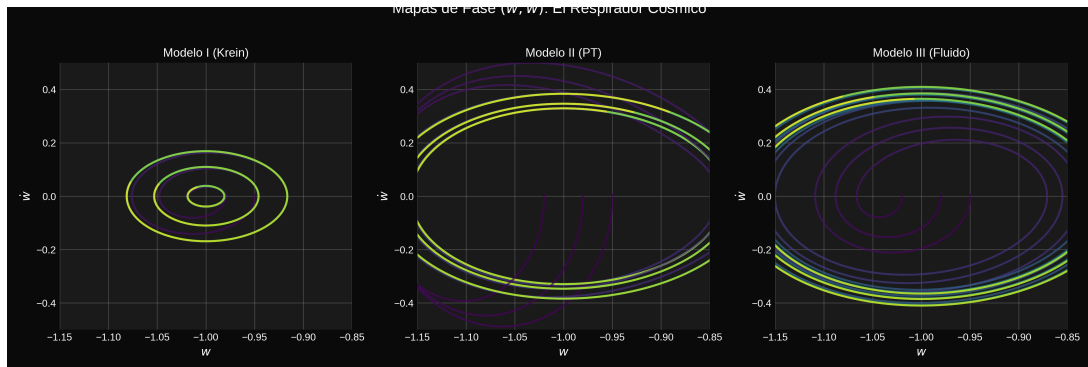
Figura 2: Mapas de fase (w, \dot{w}) para los tres modelos. Las trayectorias con gradiente de color muestran la evolución temporal. El Modelo II presenta órbitas más cerradas (resonancia), mientras que el Modelo III exhibe órbitas más amplias (memoria retardada).
