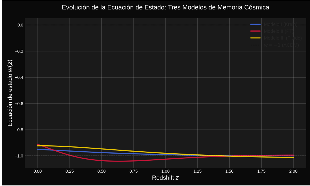
Figura 1: Evolución de la ecuación de estado w(z) para los tres modelos de memoria cósmica. Las oscilaciones reflejan la interacción entre memoria ( \tau ), disipación geométrica ( 3H ) y la temperatura del horizonte ( T_{GH} ).
